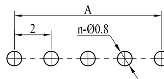
PCB 安装尺寸图
