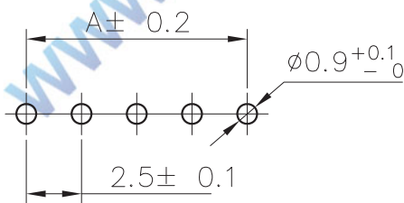
P.C.B LATOUT
