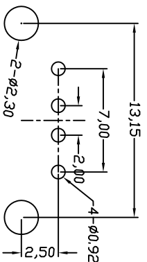
P.C.B. Layout
