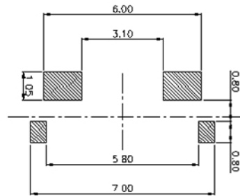
PCB. 焊接图
